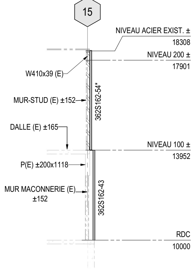
28 COUPE S302 1 : 100
