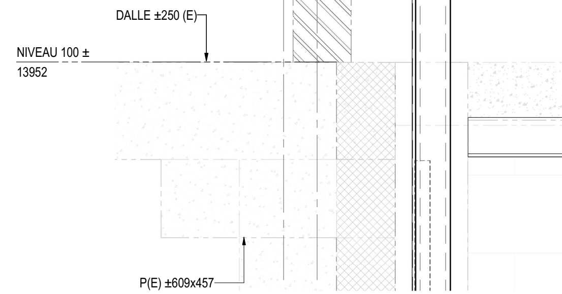
16 DÉTAIL S401 1:10
