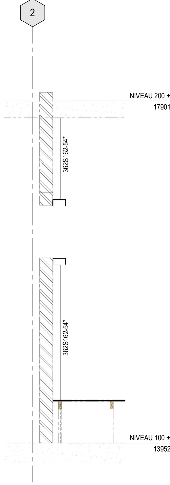
33 COUPE S202 1 : 25
