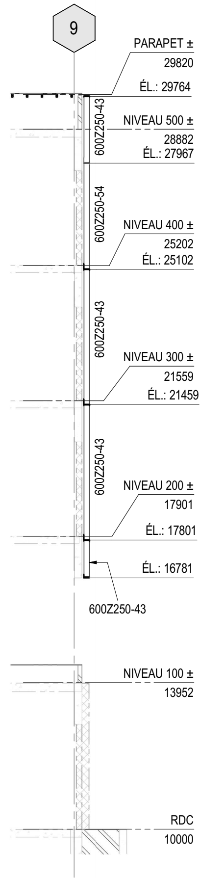
27 COUPE S201 1 : 100
