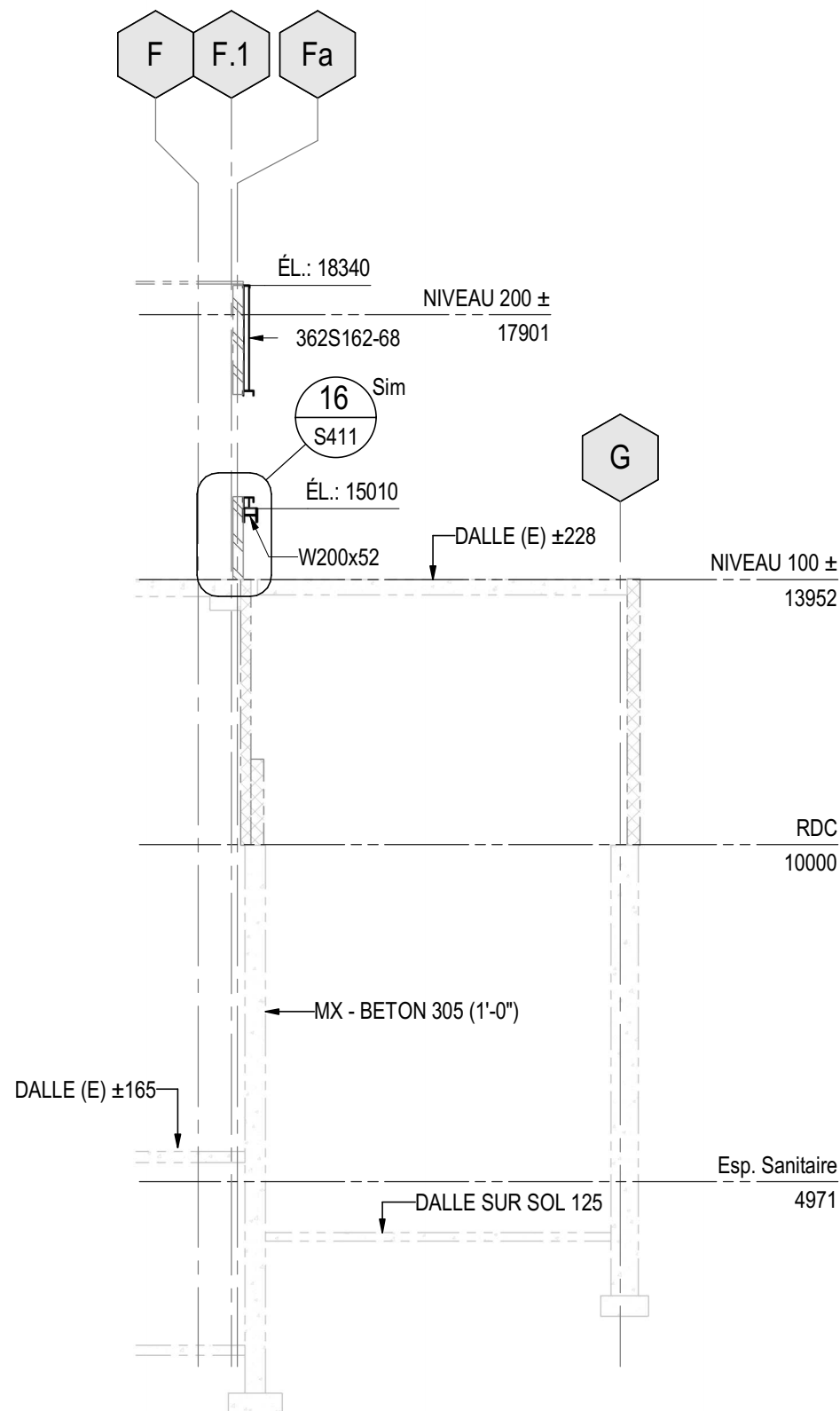
34 COUPE SAUT-DE-LOUP S201 1 : 100
