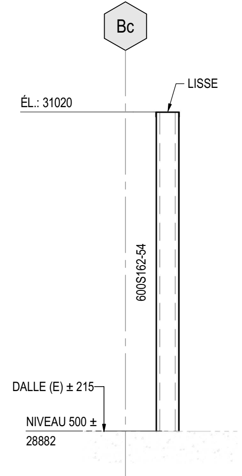
28 COUPE S302 1 : 100
