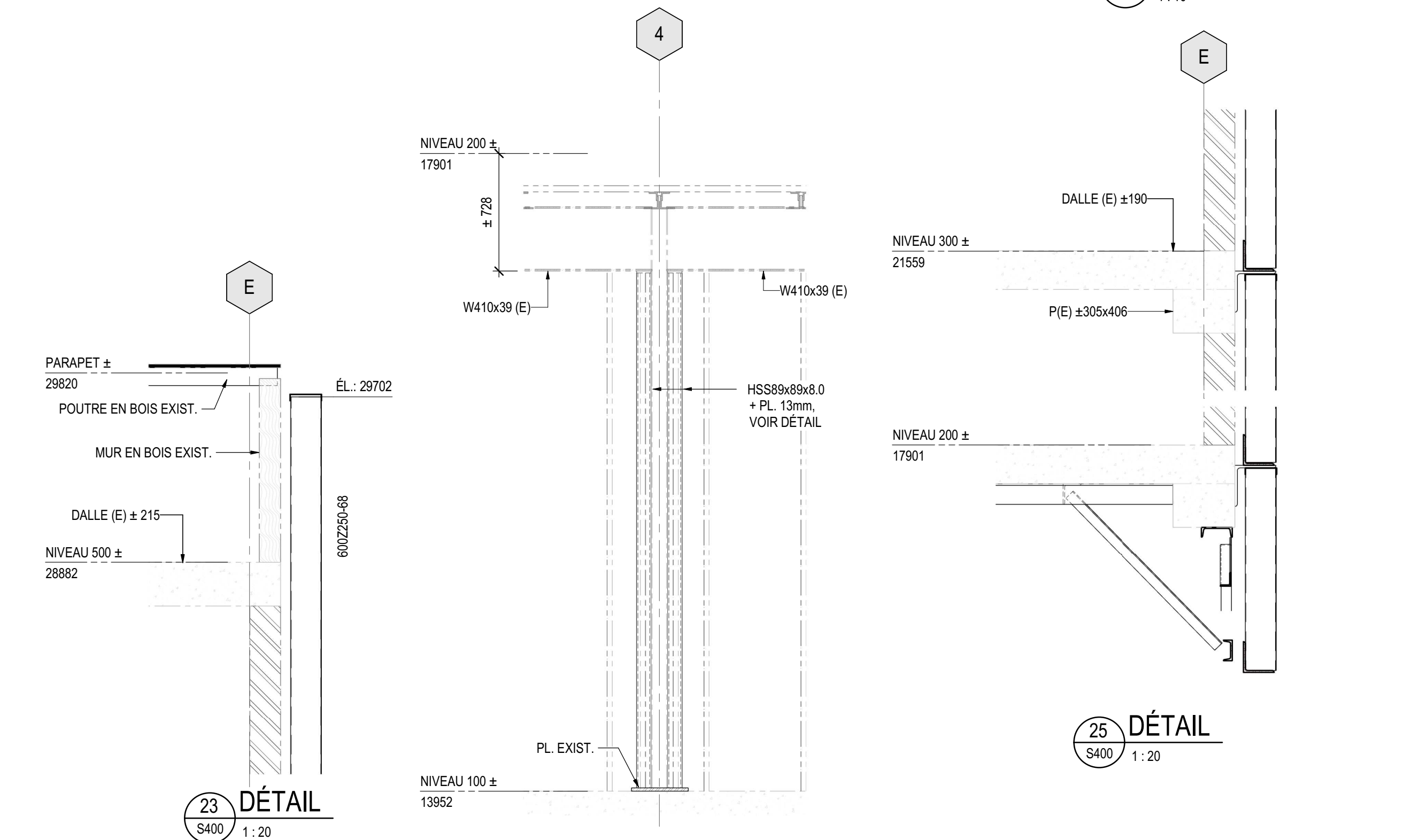
23 DÉTAIL S400 1:20
