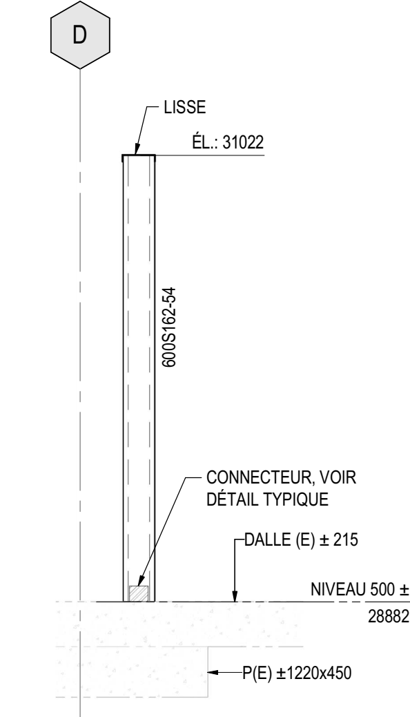
31 COUPE S300 1 : 25
