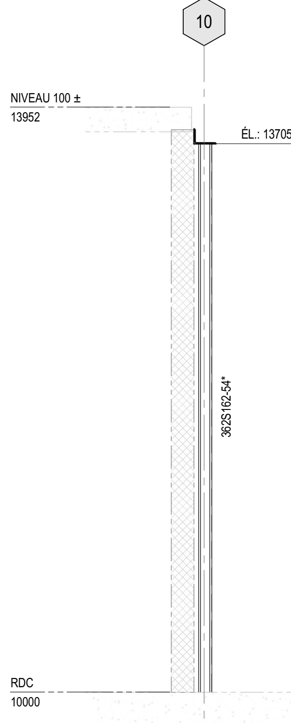
32 COUPE S201 1 : 25
